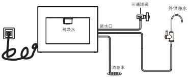
打开进水球阀
