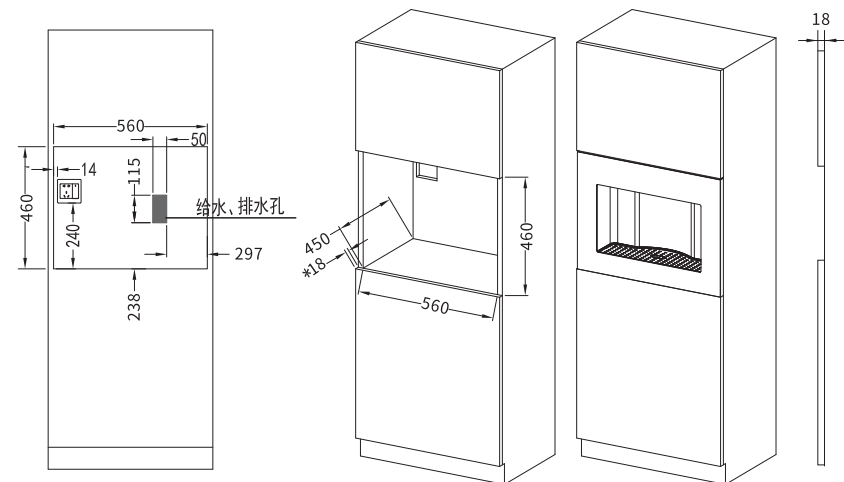
全嵌开口尺寸方式二(面板高度455)
