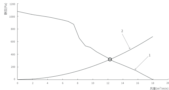
空气性能特性曲线及阻力曲线
