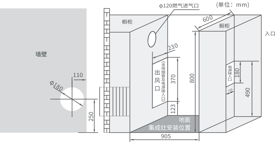
集成灶尺寸示意图 (图片仅供参考)
