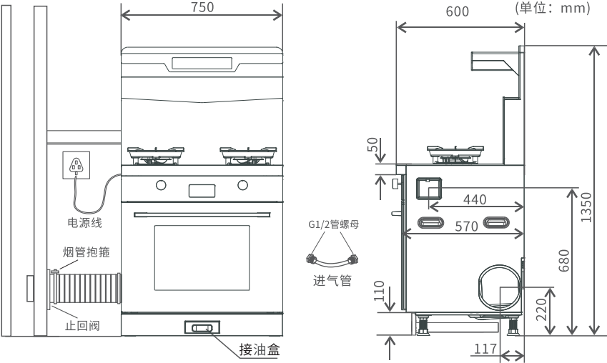
集成灶安装尺寸示意图(不同的测量方法存在细微差异，请以实际产品为准)
